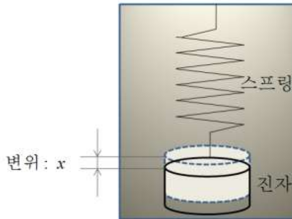
그림 2. 가속도계에 의한 비력의 측정에 활용되는 스프링 댐퍼의 원리
