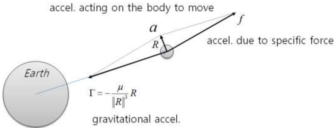
그림 4. 중력장 가속도, 비력 가속도, 그리고 운동 가속도 사이의 관계
