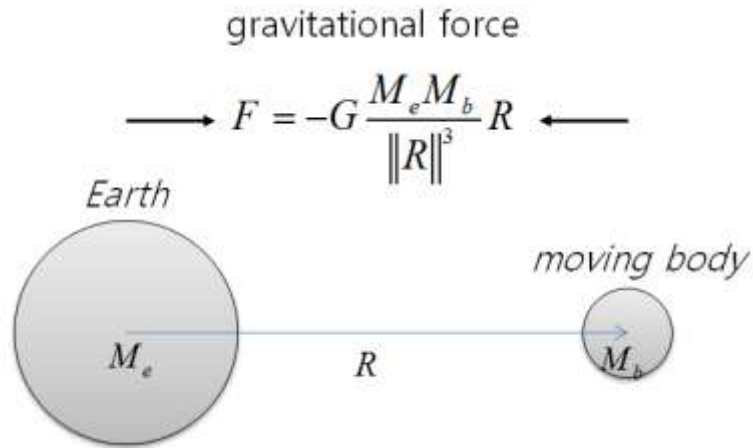
그림 1. 중력장 인력 (만유인력)의 개형
