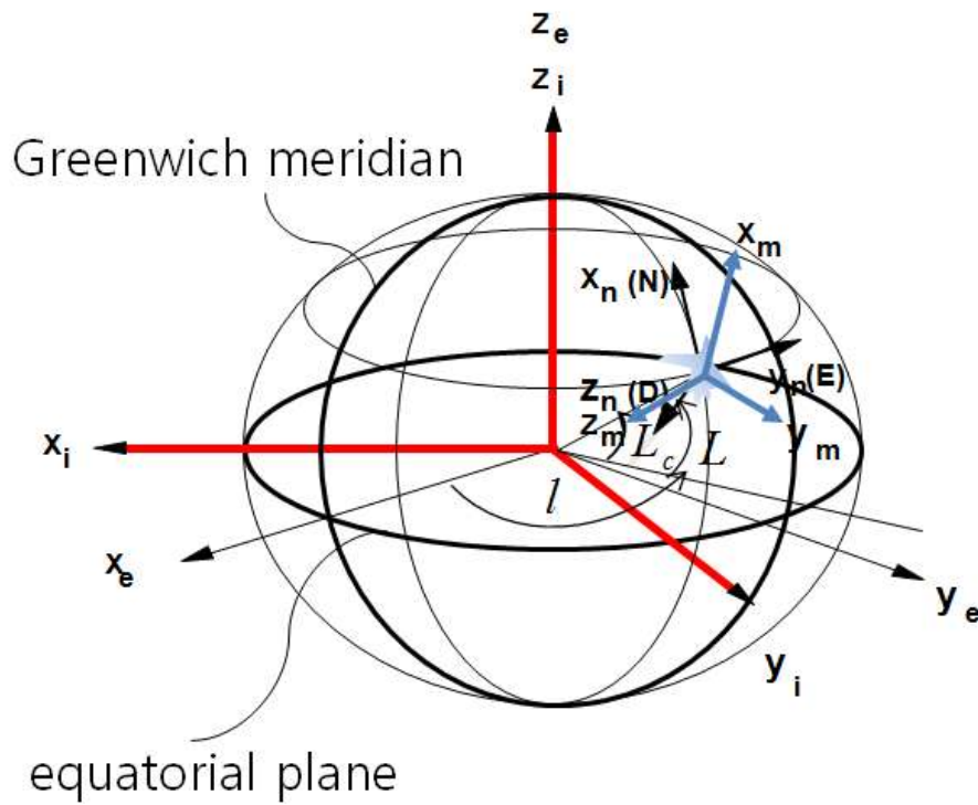
그림 3. 다양한 좌표계의 기저 벡터 개형
