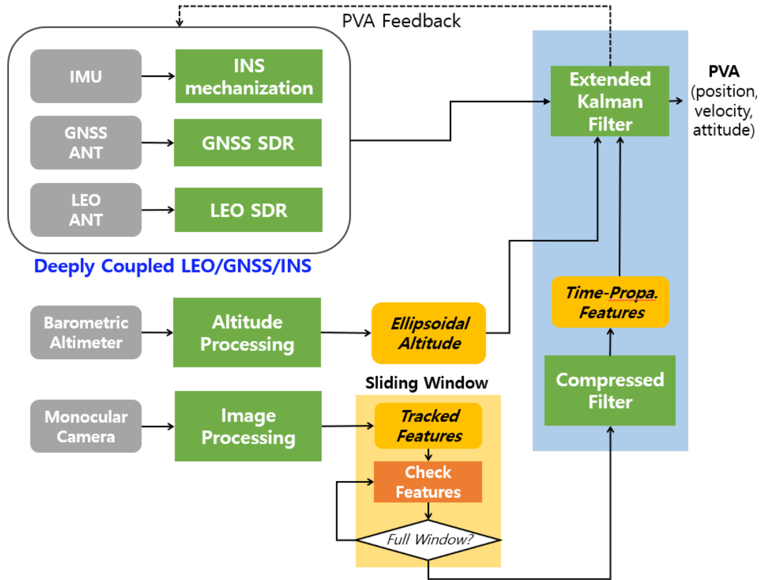
심층결합 LEO/GNSS/INS에 기반한 복합항법 시스템의 개형
